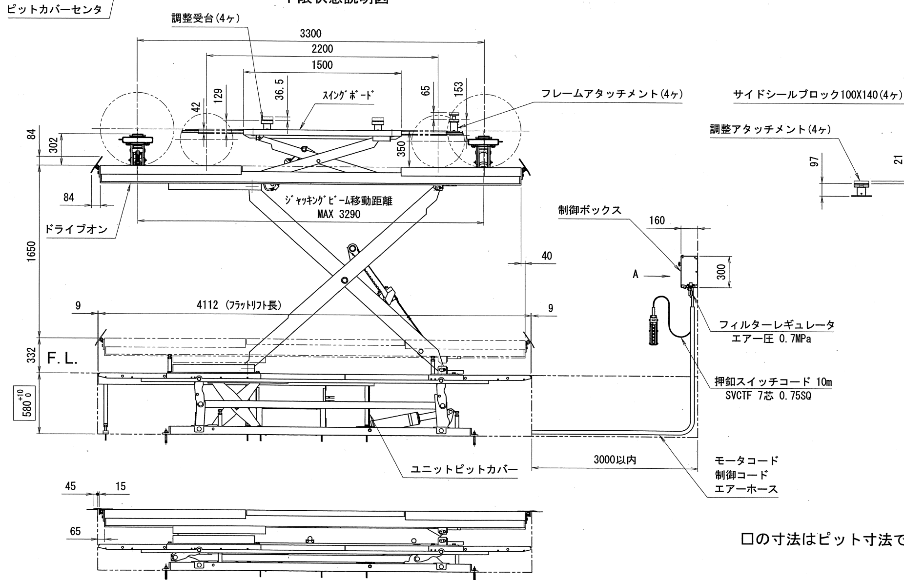
リフト収納状態説明図
