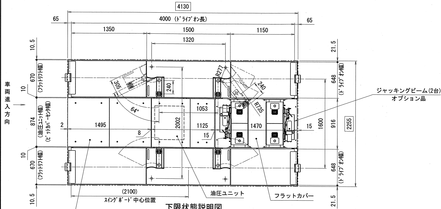
下限状態説明図
