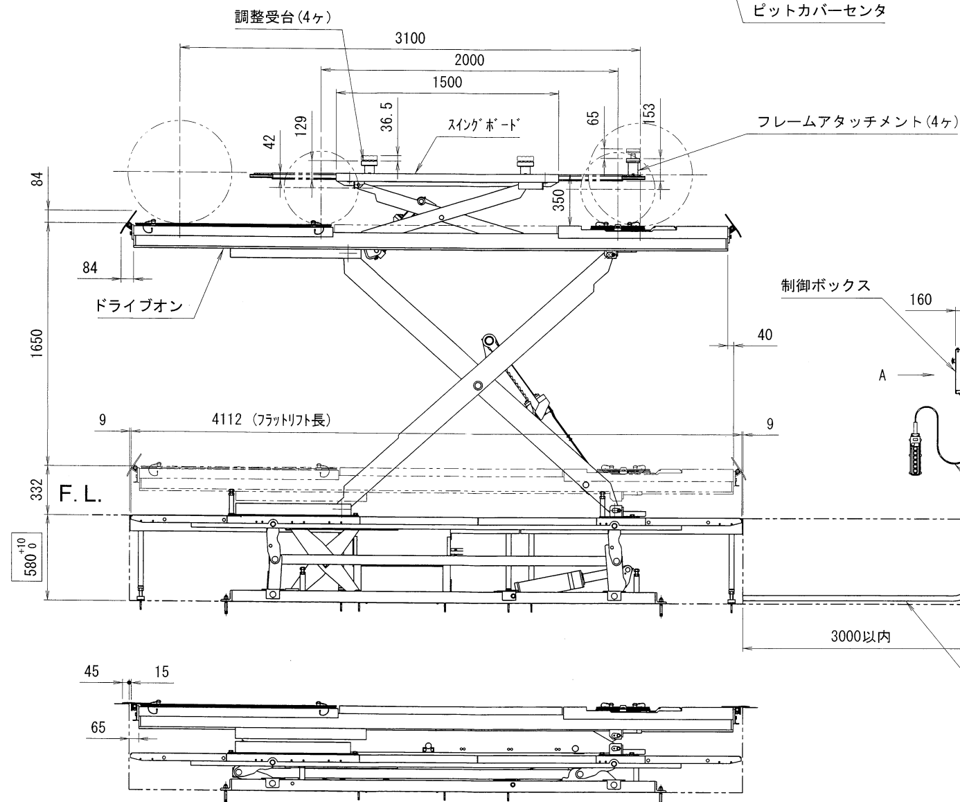
リフト収納状態説明図
