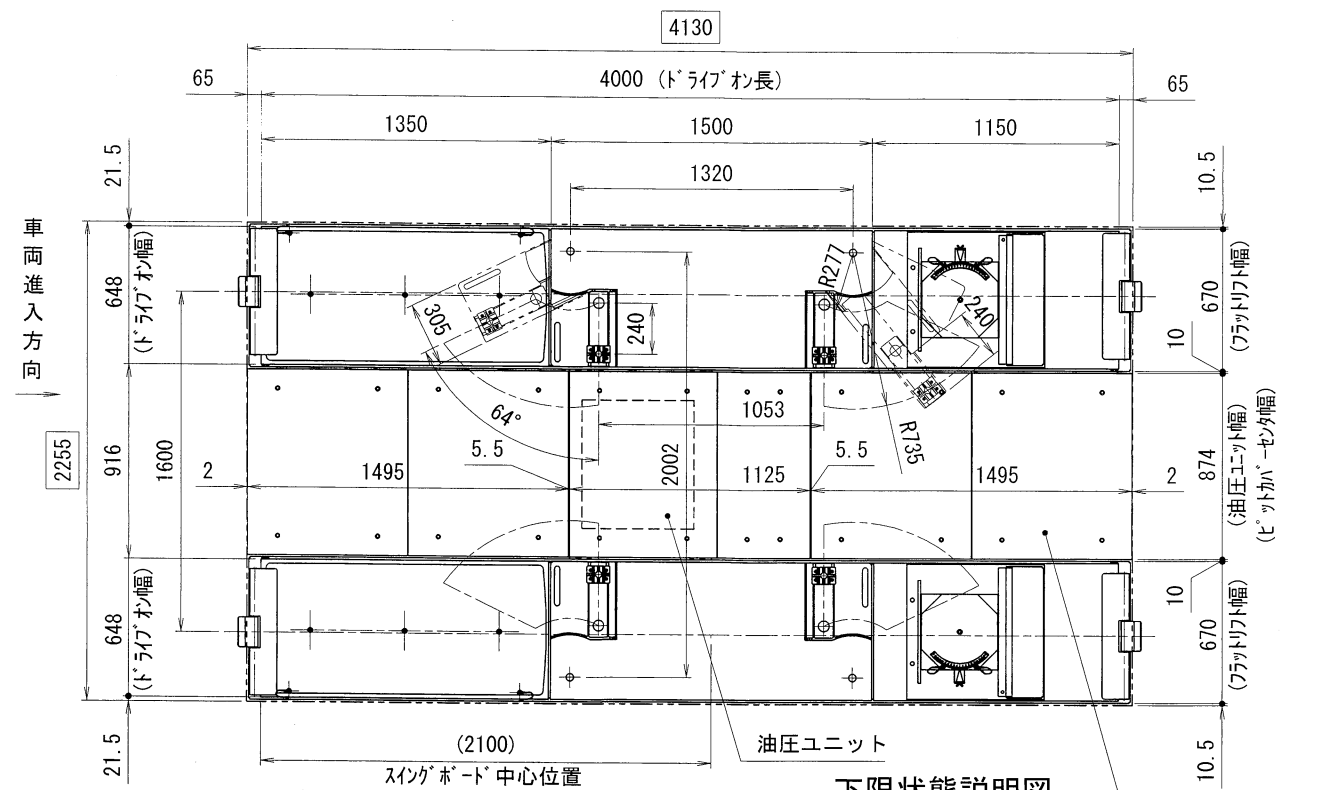
下限状態説明図
