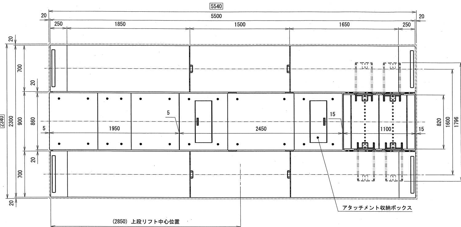
下限状態説明図
