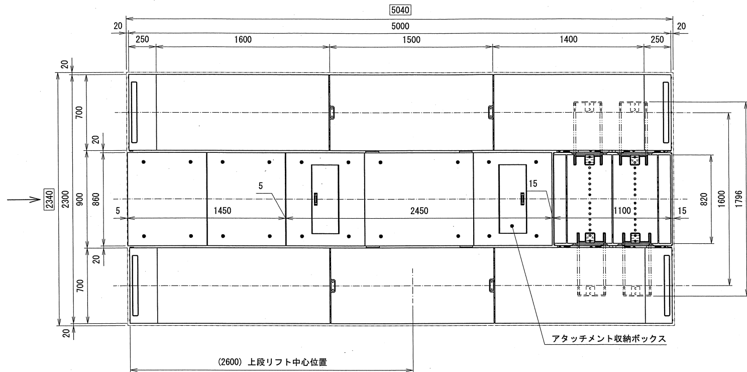
下限状態説明図
