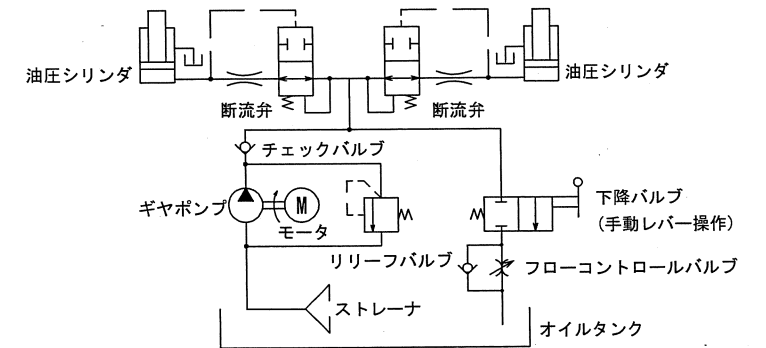
油圧回路図
