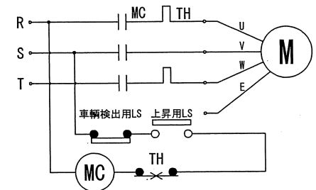
電気回路図
