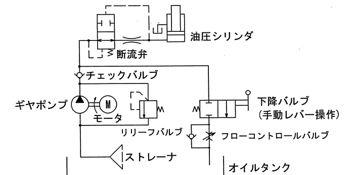
油圧回路図
