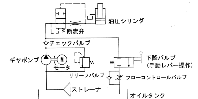
油圧回路図
