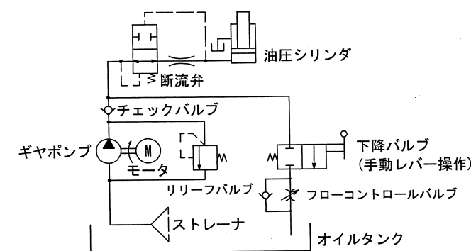
油圧回路図
