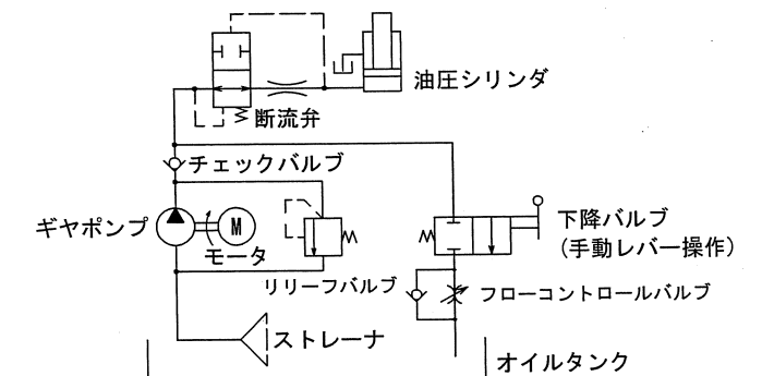
油圧回路図
