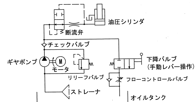
油圧回路図
