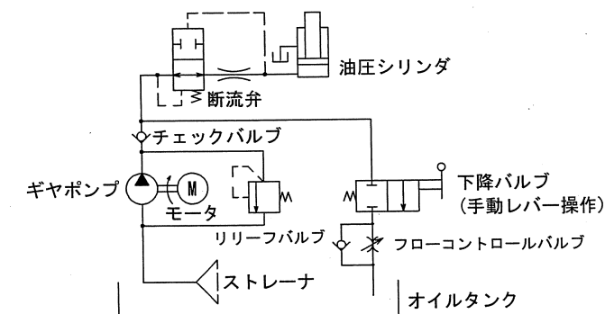
油圧回路図
