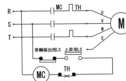
電気回路図
